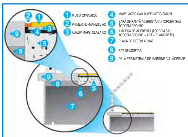
Detaliu: rost între dalele perimetrice și placile ceramice
